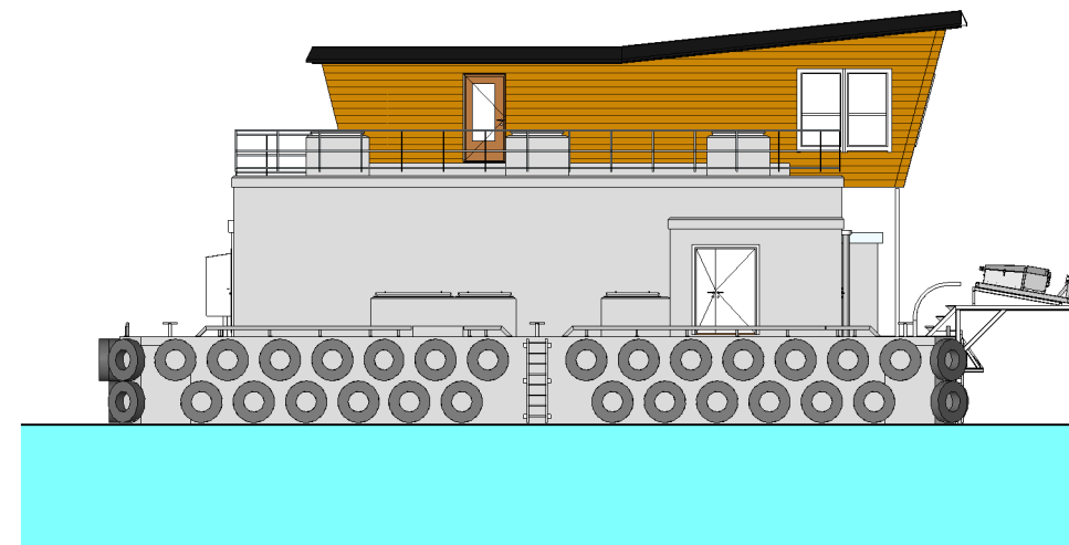
4 FASADE SILOER 1 : 200
